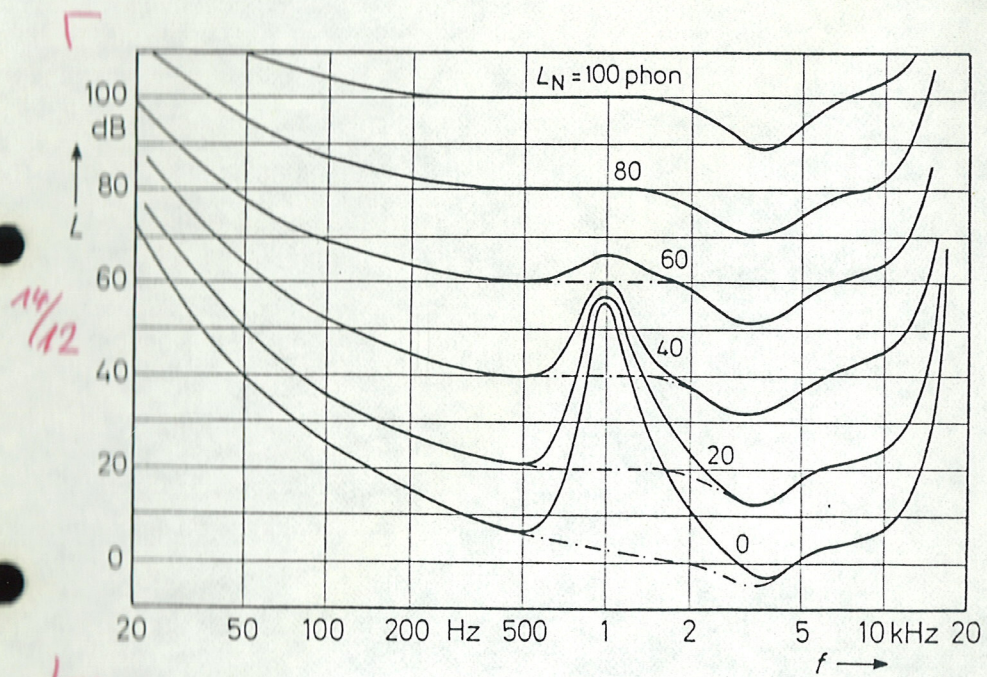
Fig. 2 Kurven gleicher Lautstärke in der Hörfläche für das ebene Schallfeld bei Schmalbandstörerschens von 60 \text{ dB}
