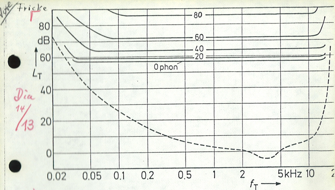
Fig. 1 Phon-Kurven bei Anwesenheit eines gleichmäßig verdeckten Störerschens von 60 \text{ dB} / \Delta f_G (bei f \leq 500 \text{ Hz} )
