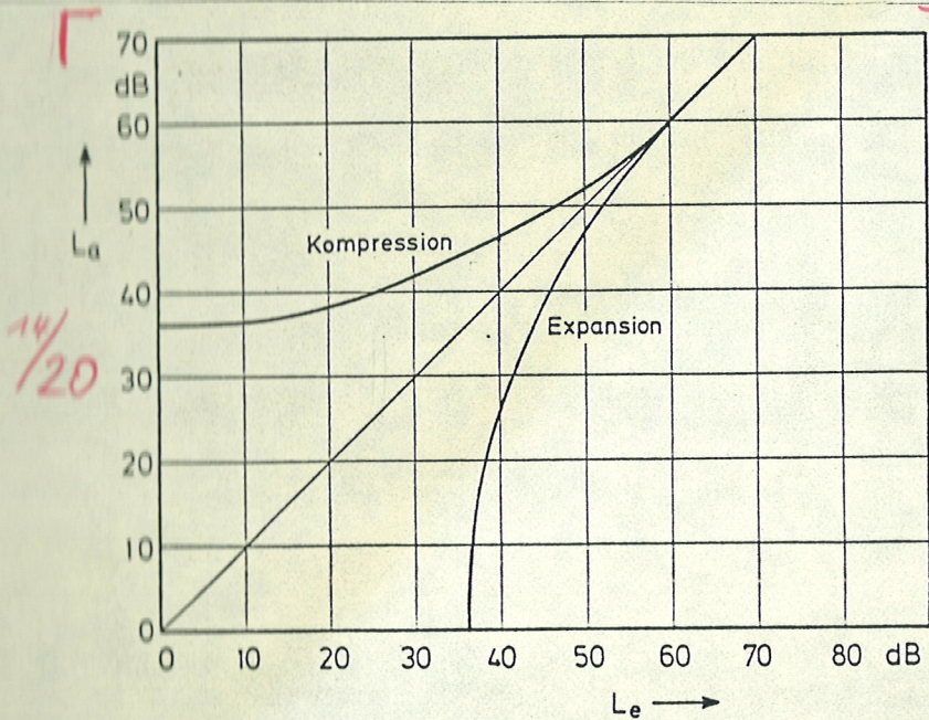
Fig. 8 Expansionskurve des Gehörs für einen durch 40 \text{ dB} / \Delta f_g Schmalbandrauschen gedrosselten 1 kHz-Ton (nach ZWICKER 1963)
