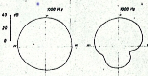
Abb. 5 Polardiagramme zweier Geigen bei 1000 Hz (Stegebene)
