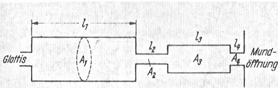
Annäherung des Ansatzrohres durch vier zylindrische Röhren nach DUNN
