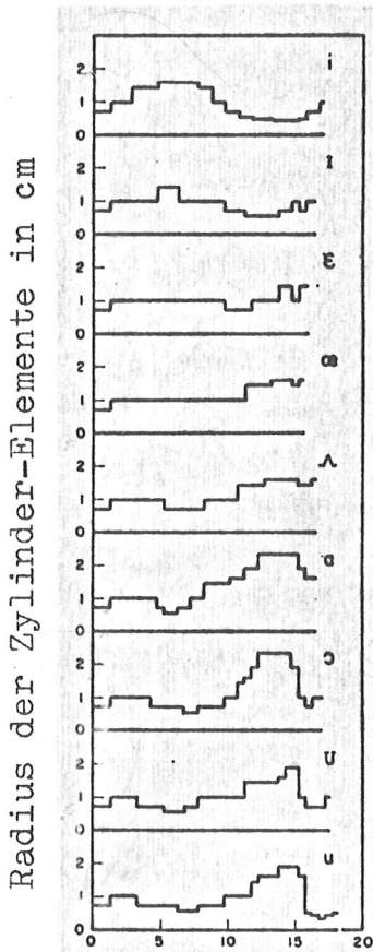
Abstand von der Glottis (cm)
