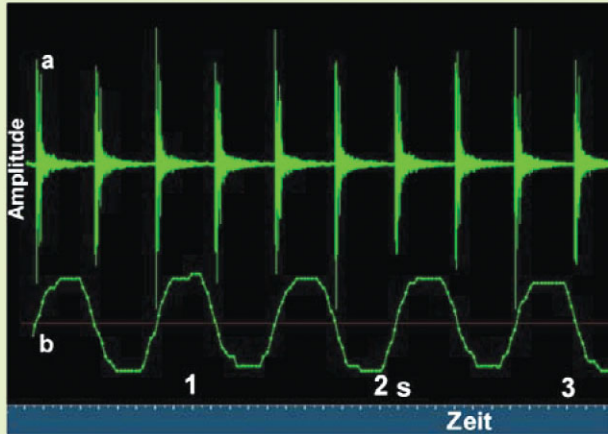
ABB. 3 SYNCHRONISATIONSPROZESSE
