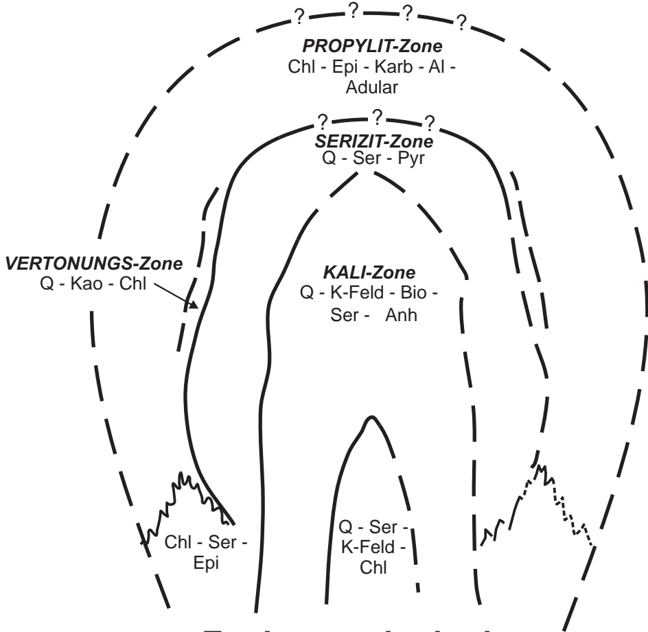
Zonierung der hydrothermalen Alteration
