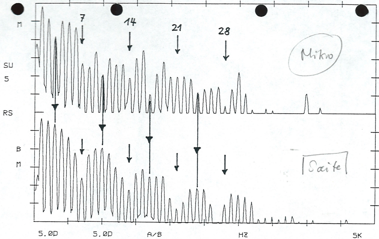
Bild 4: Spektrum des abgestrahlten Schalles (Mikrophonaufnahme, oben) und der Saitenschnelle an der Anstrichstelle (bei ca. 1/7 Saitenlänge, unten) von der G-Saite des Kontrabasses (100 Hz) Abstrich.
